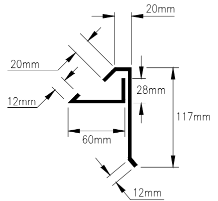
BARGE COVER DETAIL N.T.S.
