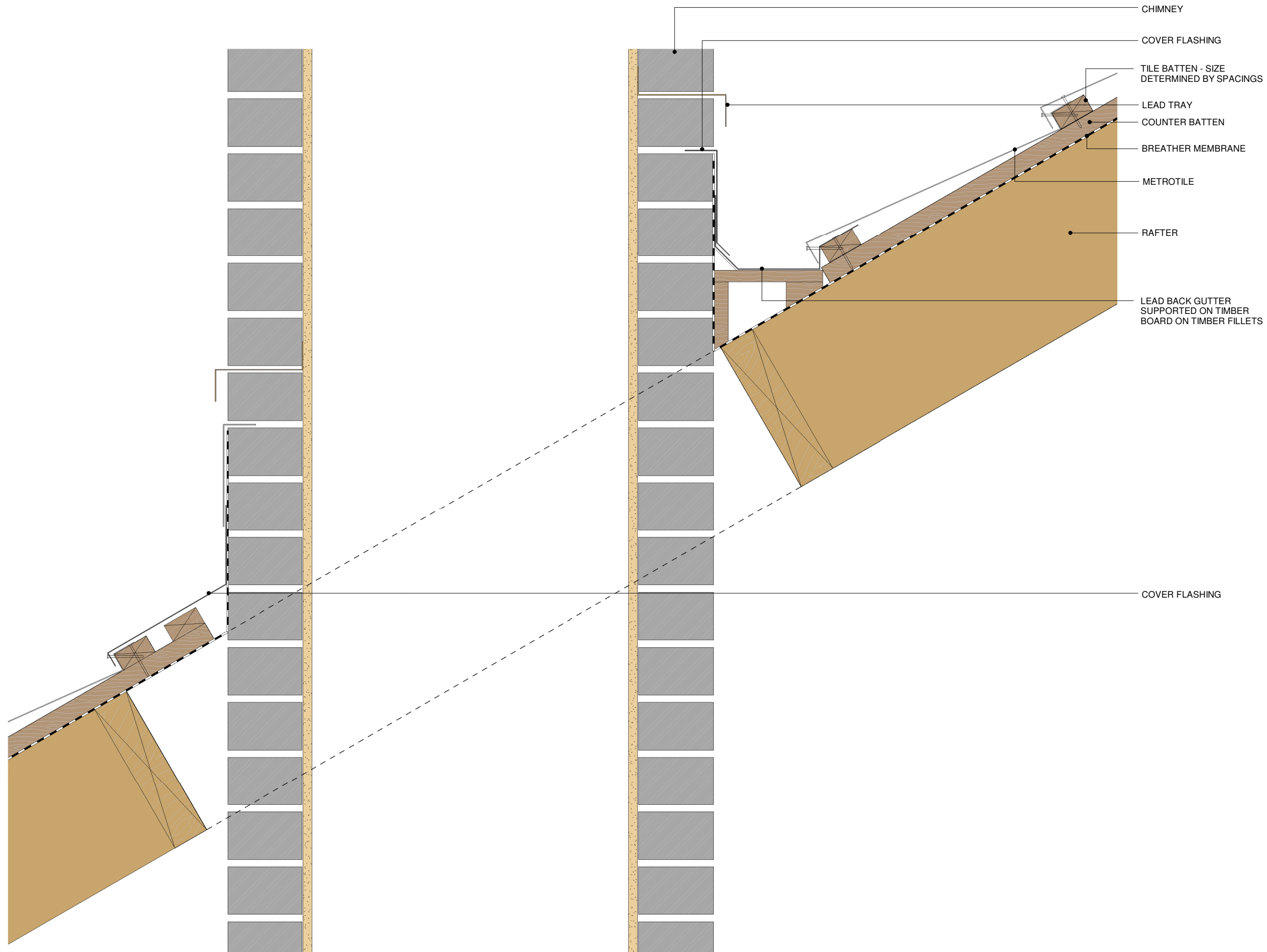
1 Metrotile Chimney Detail 1 : 5
